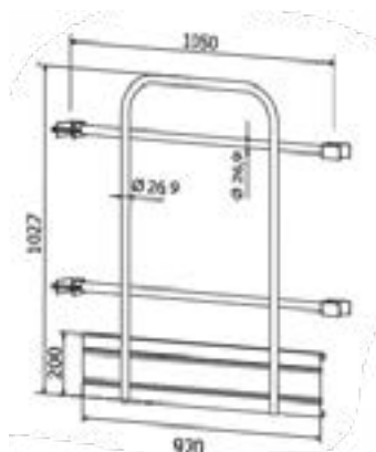
Cancelletto di testata
