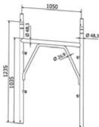
Mezzo telaio
