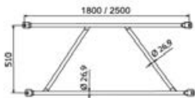
Spondina di facciata
