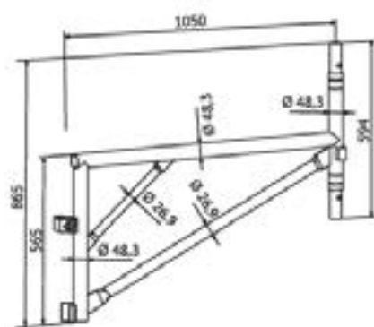
Mensola per disassamento da 1,05 m
