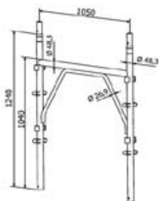
Mezzo telaio
